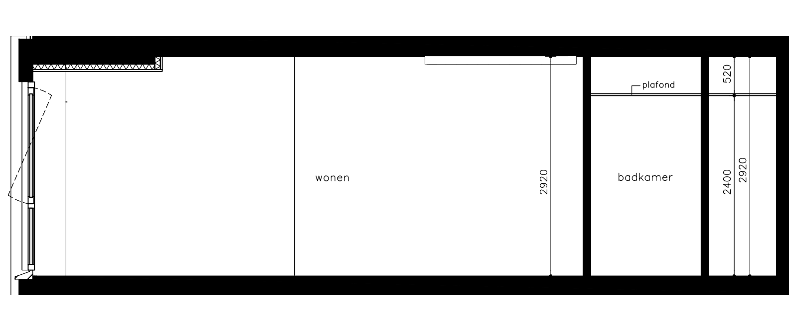
Doorsnede
