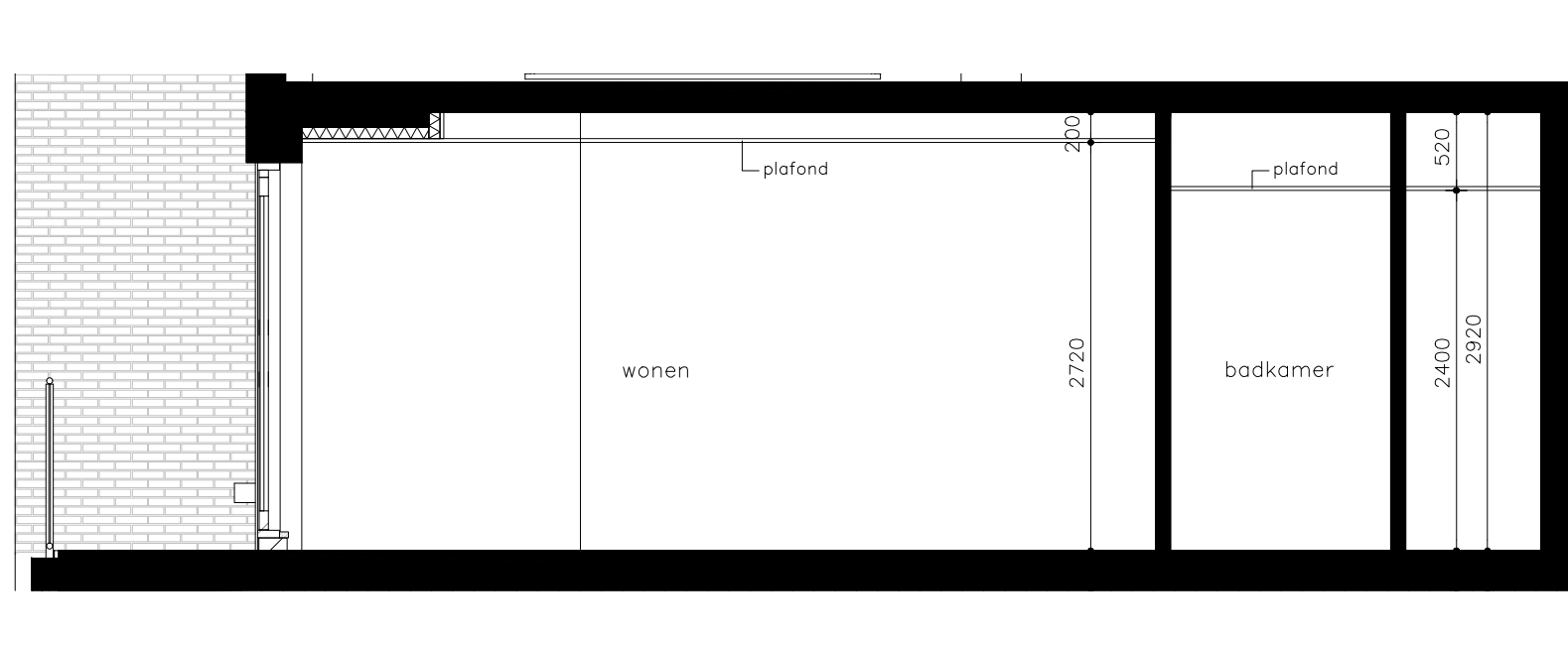
Doorsnede
